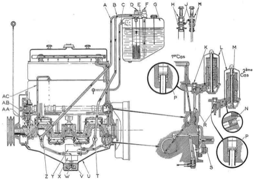
Circuit de graissage
